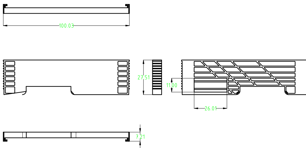
3099挡板外形尺寸
