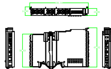
6000模块16点外形尺寸
